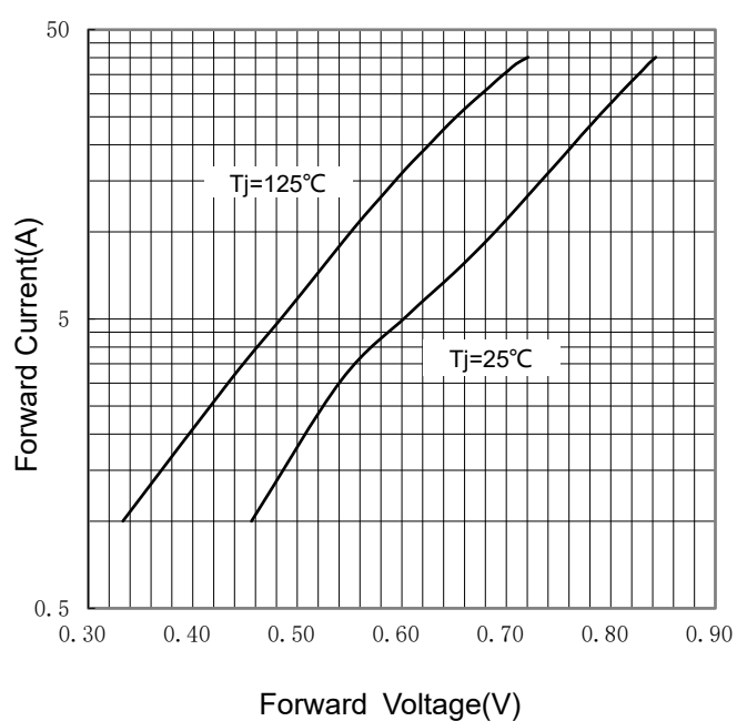
FIG 4: I_F - V_F
