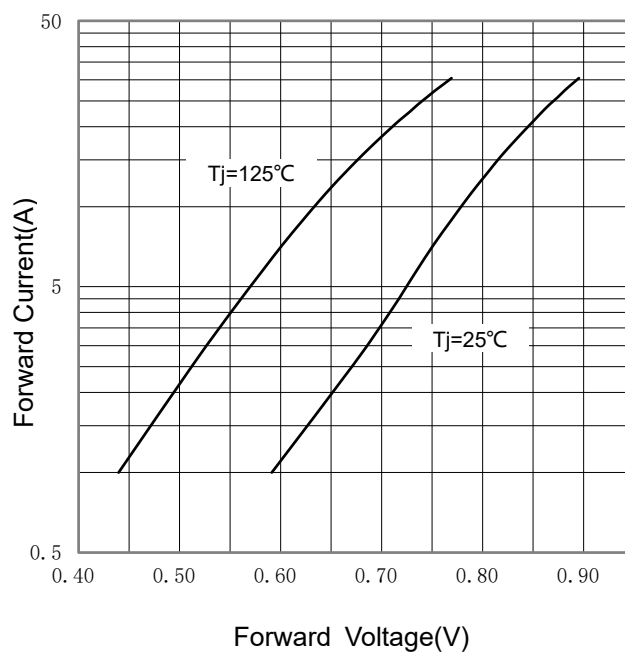
FIG 4: I_F - V_F
