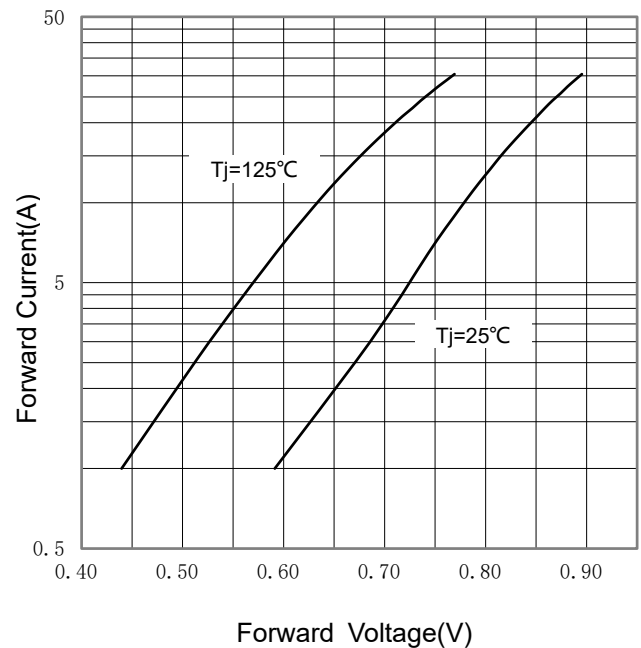
FIG 4: I_F - V_F
