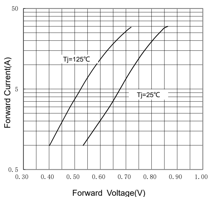
FIG 4: I_F - V_F
