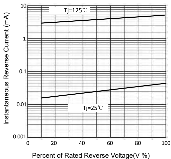
FIG 3: V_R - I_R
