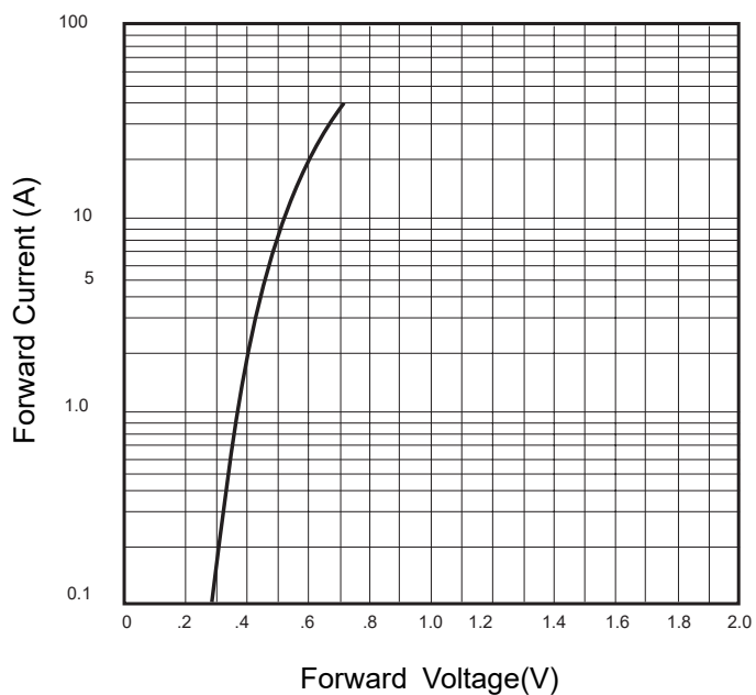
FIG 4: I_F - V_F
