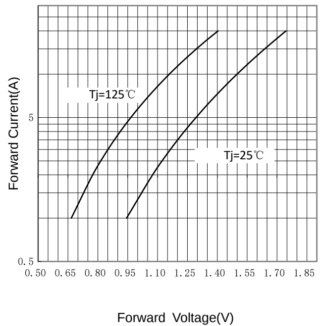
FIG 4: I_F - V_F
