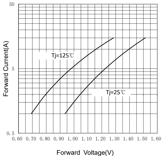
FIG 4: I_F - V_F
