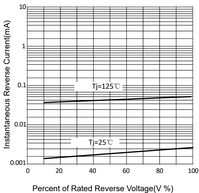
FIG 3: V_R - I_R
