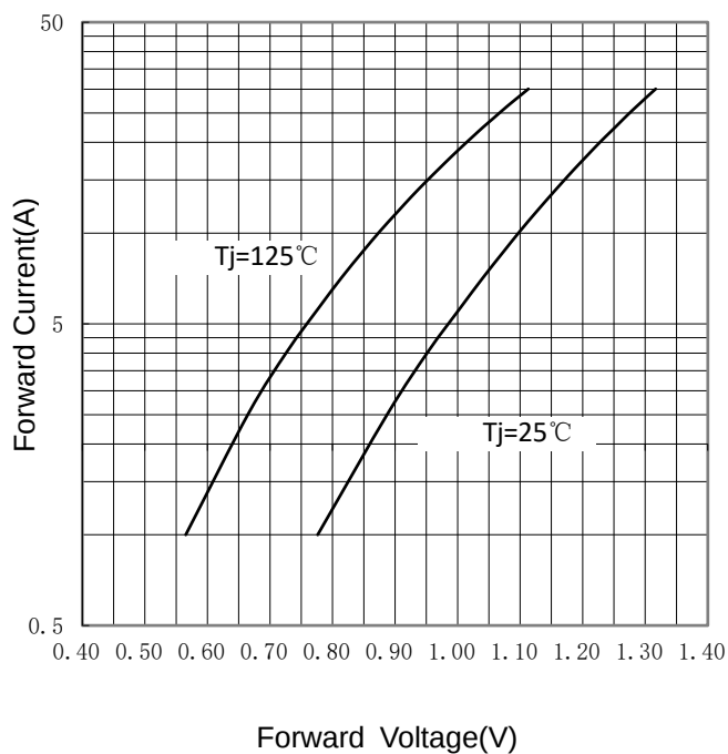
FIG 4: I_F - V_F
