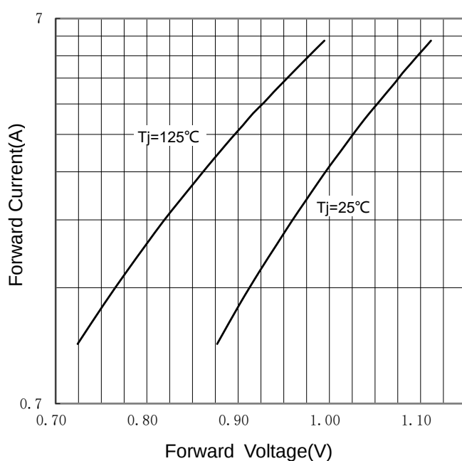
FIG 4: I_F - V_F
