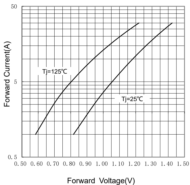
FIG 4: I F -V F
