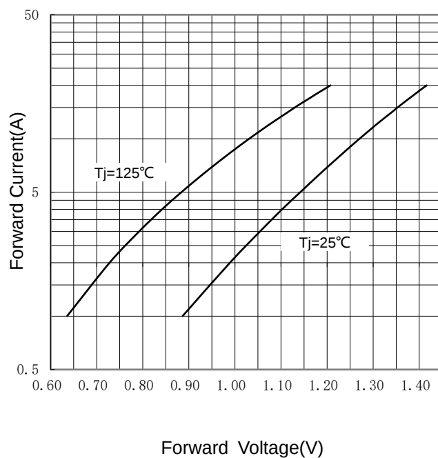
FIG 4: I F -V F
