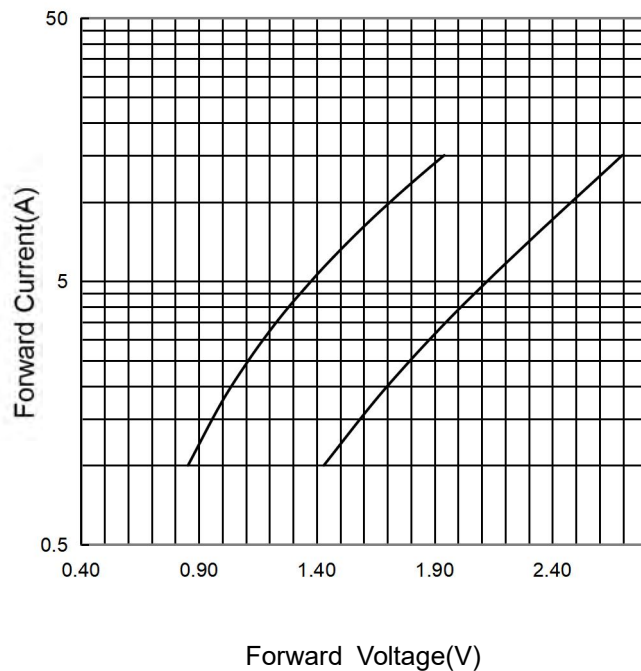
FIG 4: I_F - V_F
