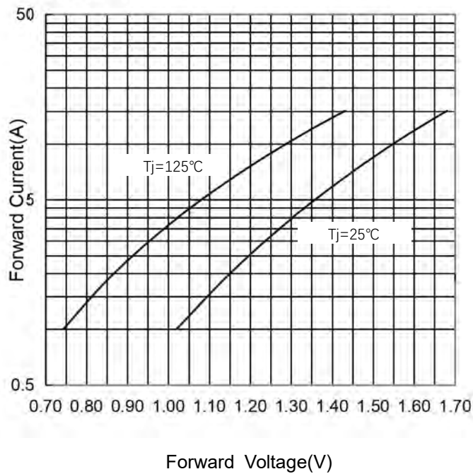
FIG 4: I_F - V_F
