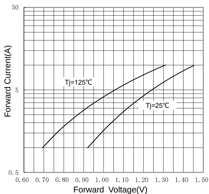
FIG 4: I_F - V_F
