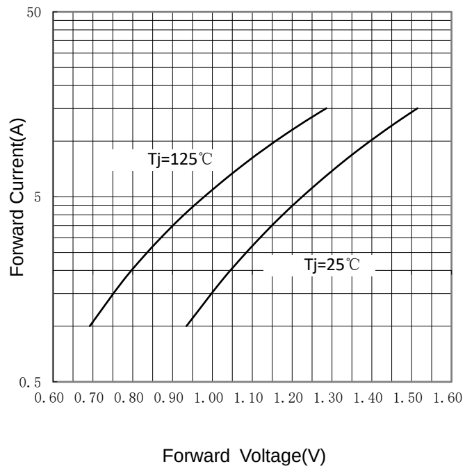
FIG 4: I F -V F
