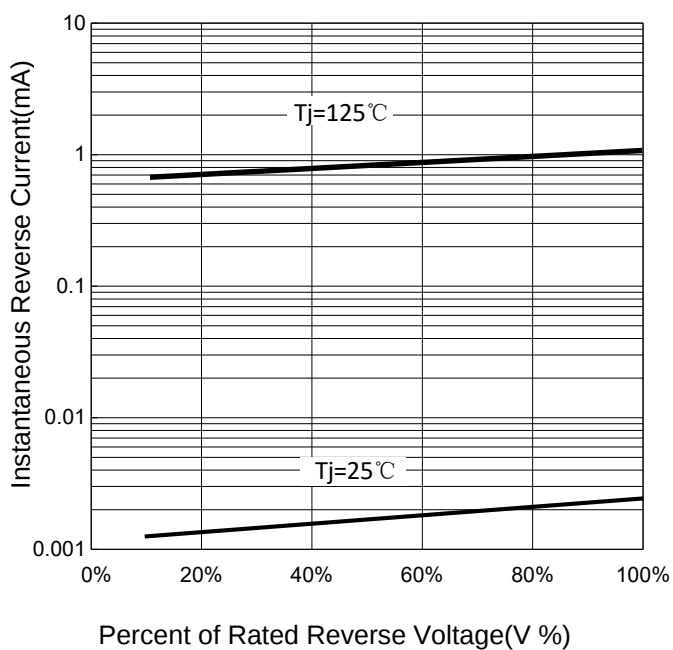
FIG 3: V_R - I_R
