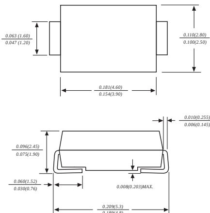
DO-214AC/SMA
