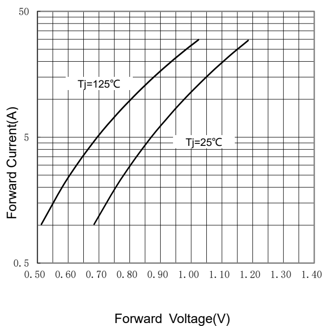
FIG 4: I_F - V_F
