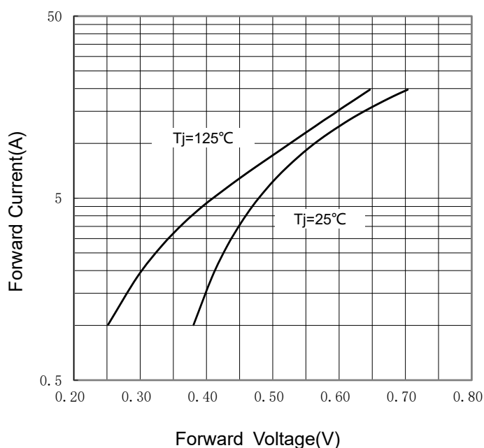
FIG 4: I_F - V_F
