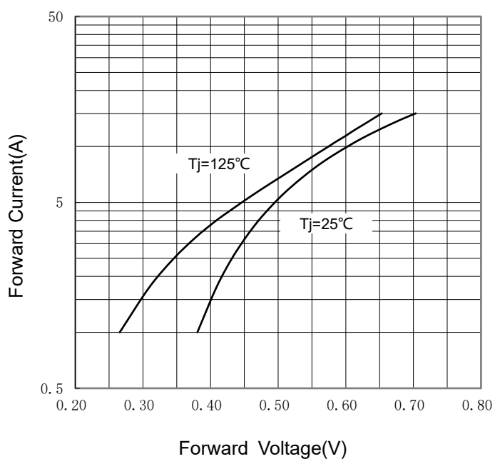
FIG 4: I_F - V_F
