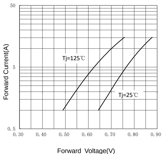
FIG 4: I_F - V_F
