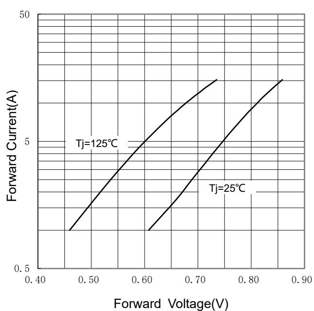
FIG 4: I_F - V_F
