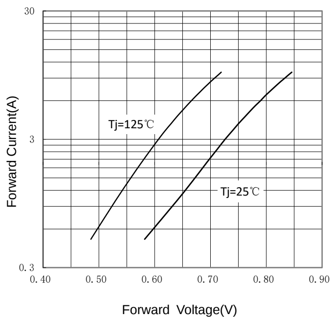
FIG 4: I_F - V_F
