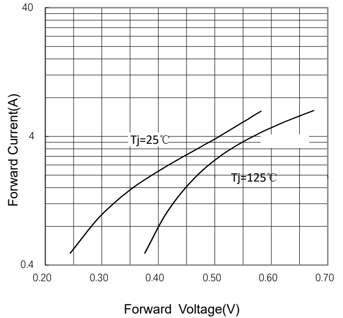
FIG 4: I_F - V_F
