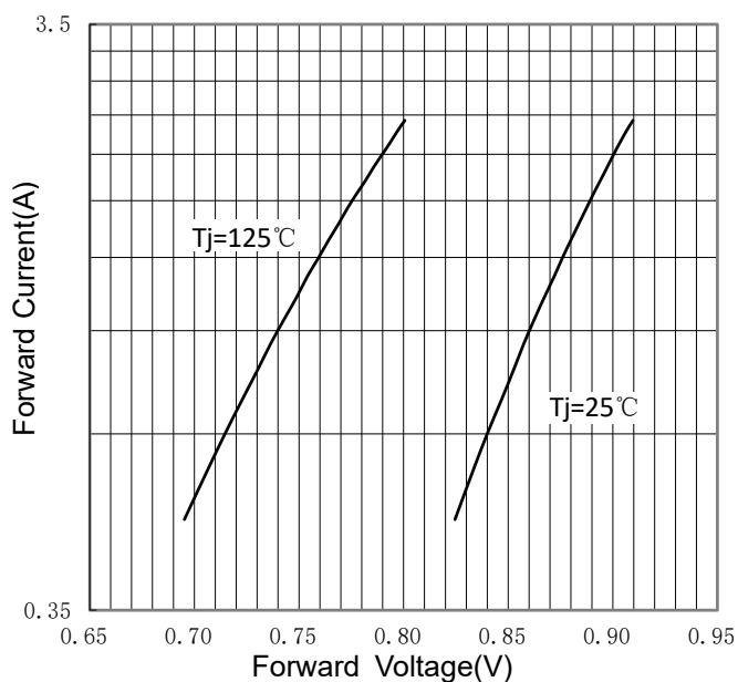
FIG 4: I_F - V_F
