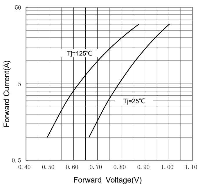
FIG 4: I_F - V_F
