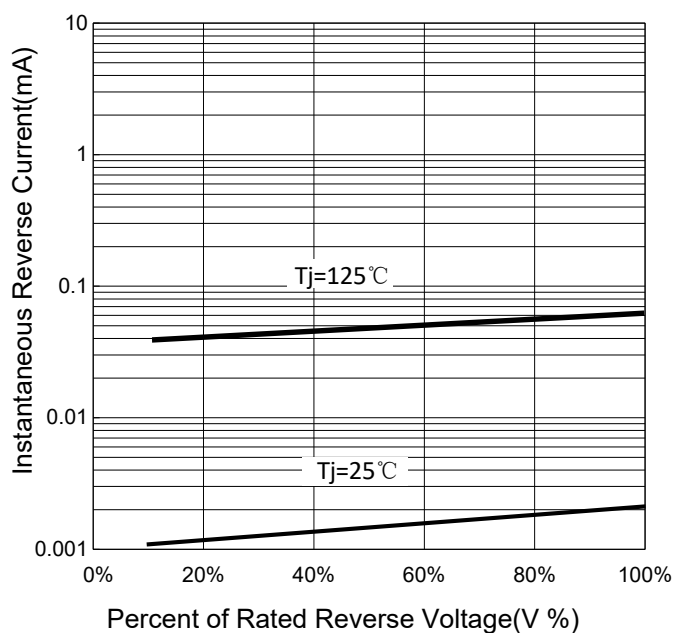
FIG 3: V_R - I_R
