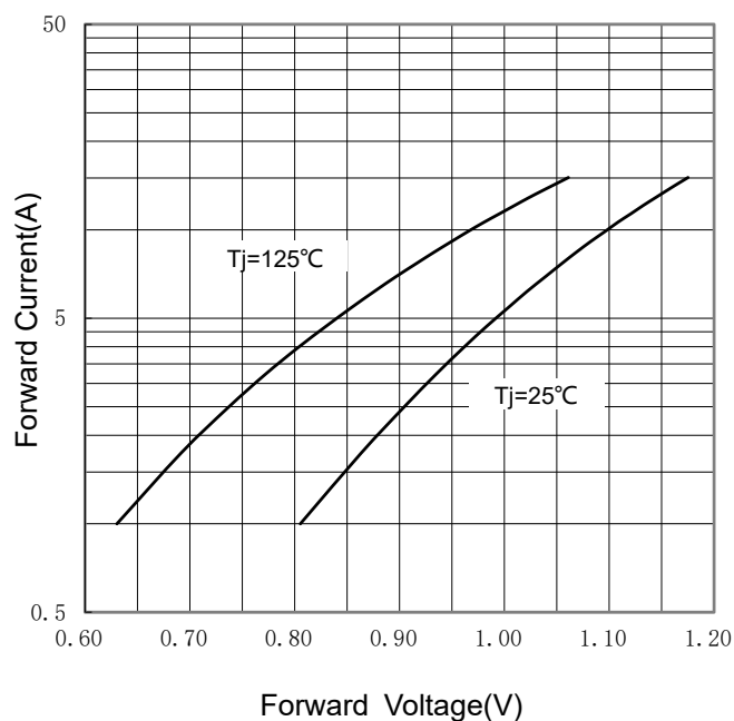
FIG 4: I_F - V_F
