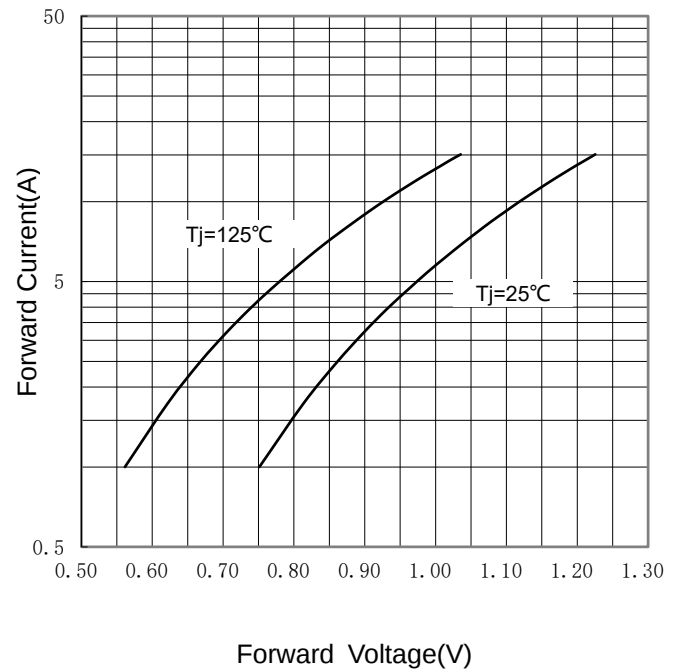
FIG 4: I_F - V_F
