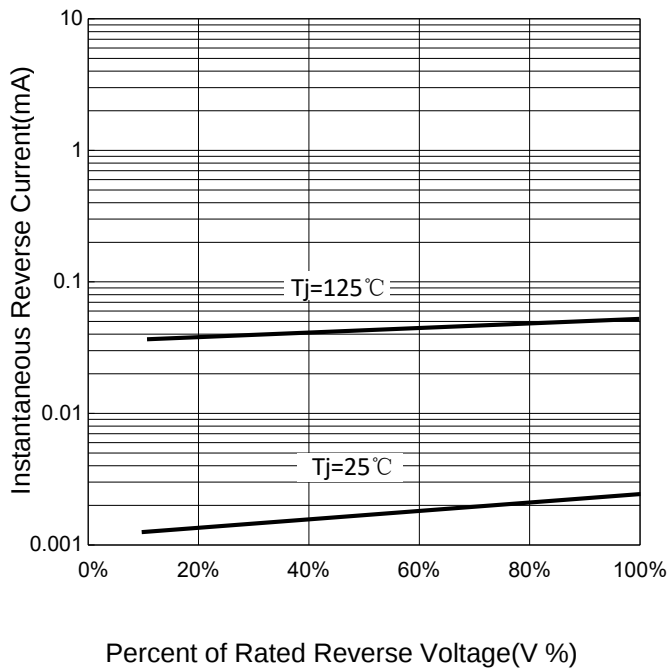
FIG 3: V_R - I_R
