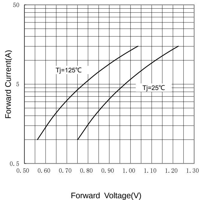
FIG 4: I_F - V_F
