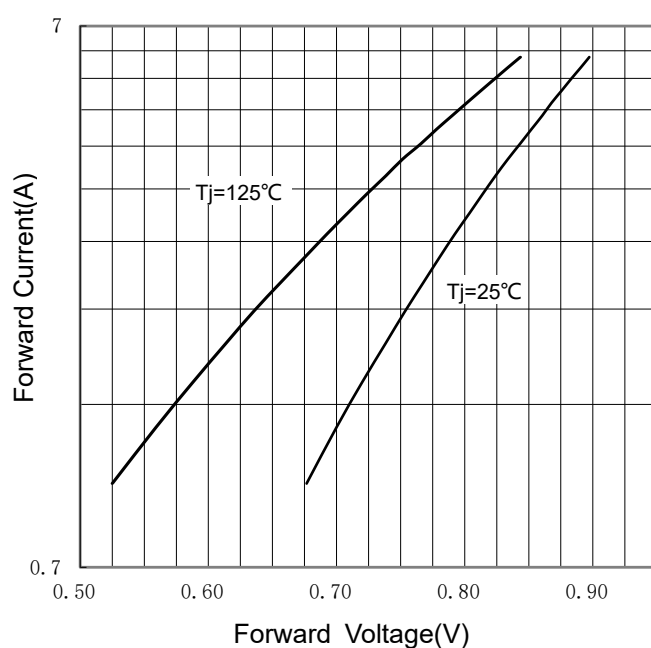
FIG 4: I_F - V_F
