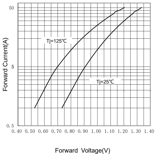
FIG 4: I_F - V_F
