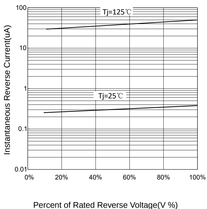
FIG 3: V_R - I_R
