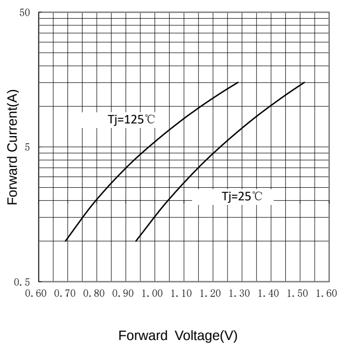
FIG 4: I_F - V_F
